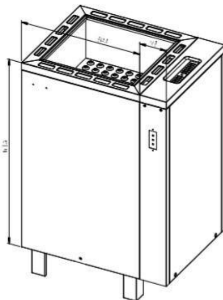
Fig.3 Dimensioni esterne
