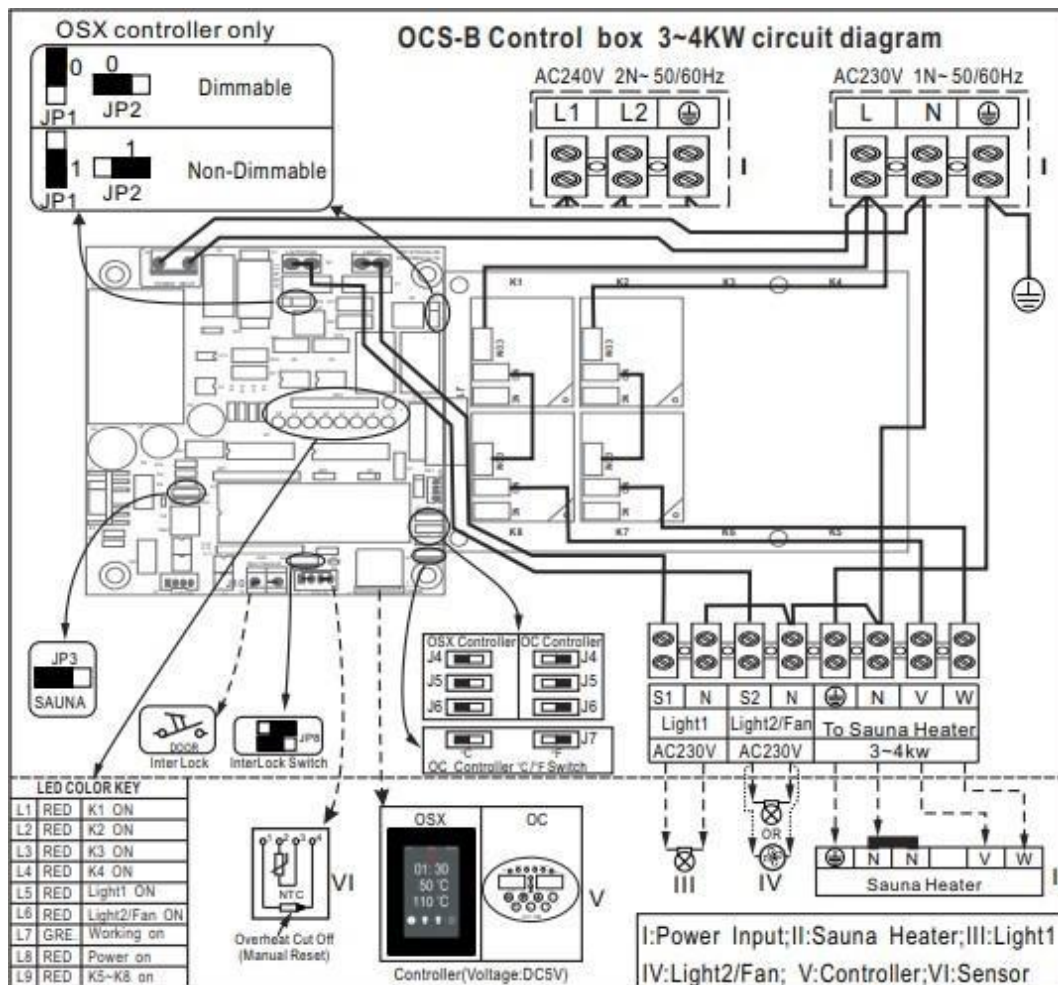
Fig 2.c - Diagramma dei circuiti per la Control Box OCSB - 3-4 kW (a partire da Maggio 2022)
